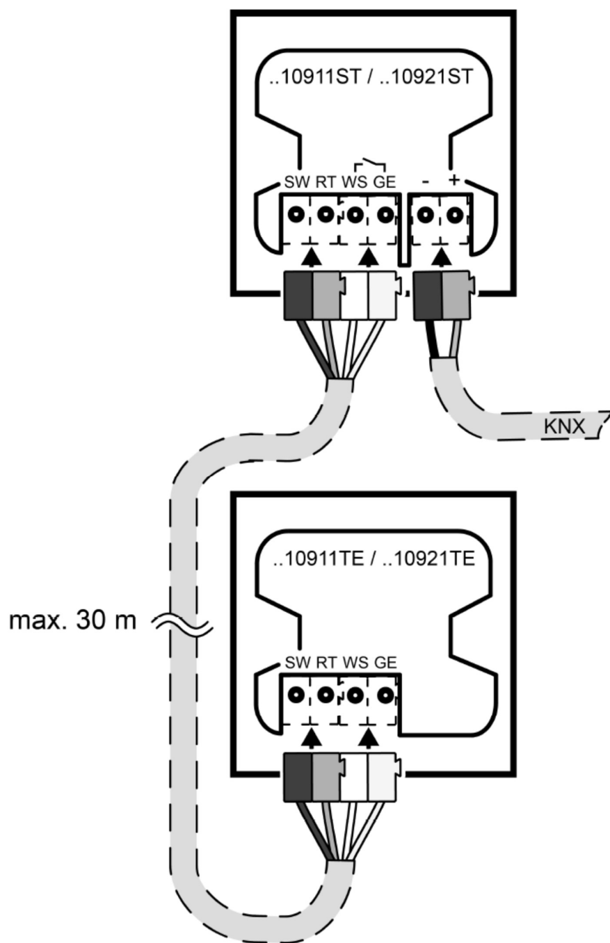
Vista trasera y conexión del módulo de ampliación
