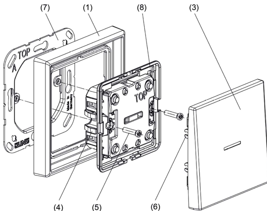
Figura 3: Despiece y montaje
