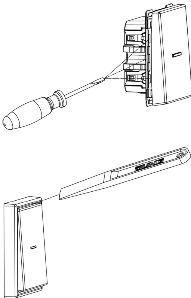
Figura 4: Posibilidades de desmontaje
