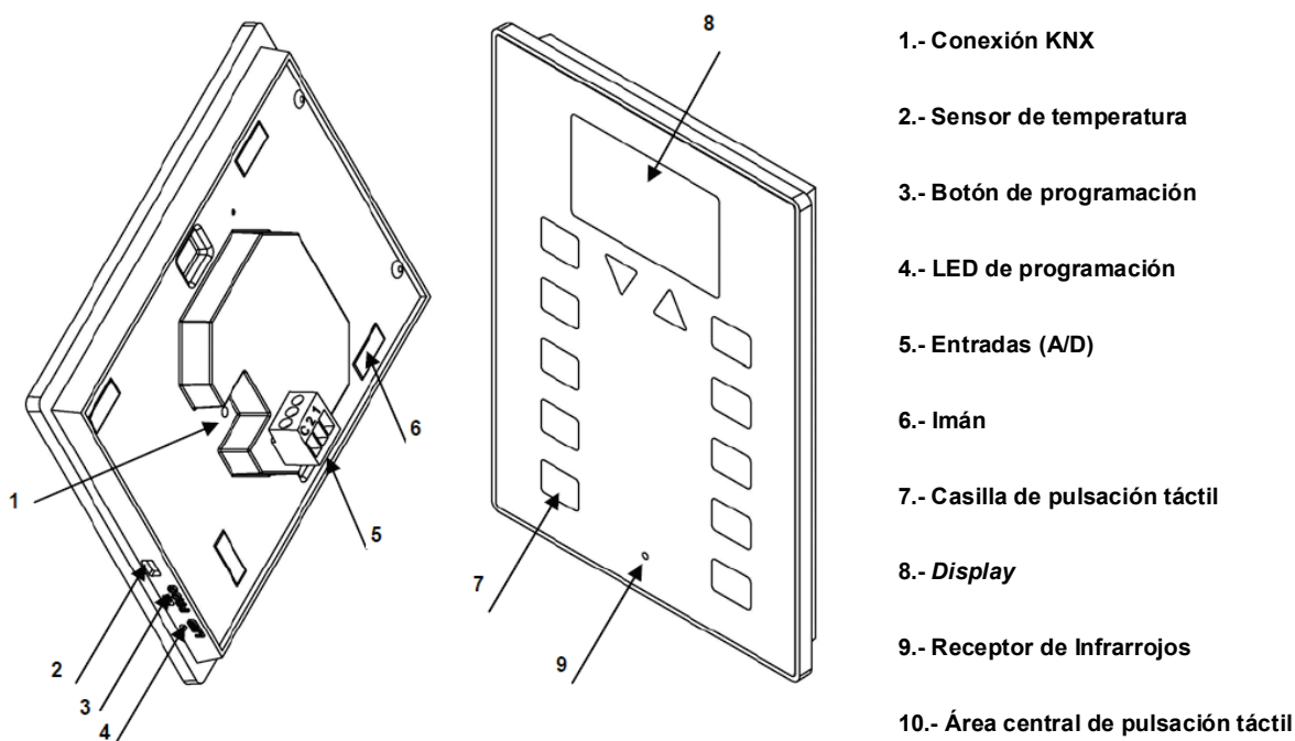
Figura 2. ZAS. Esquema de elementos.
