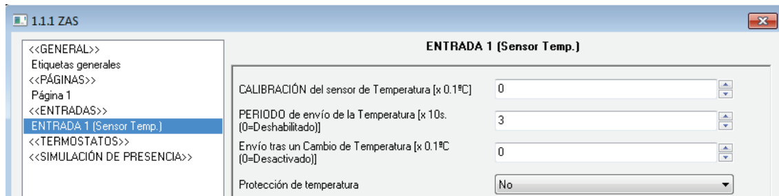
Figura 22. Entrada: sonda de temperatura
