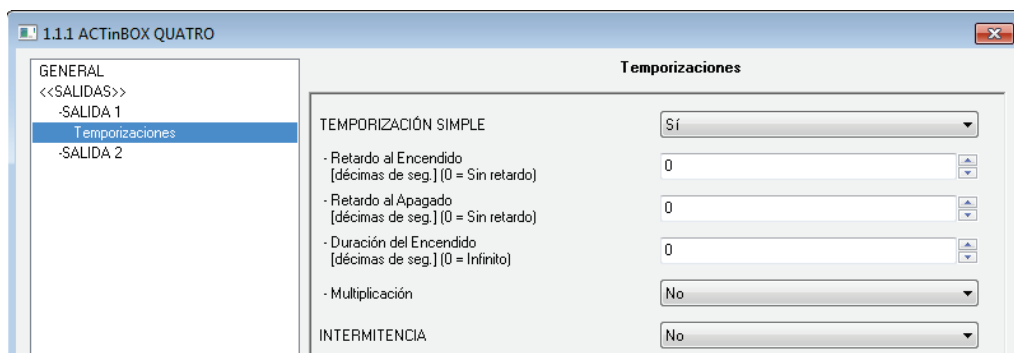
Figura 8. Pantalla de temporizaciones. Temporización simple
