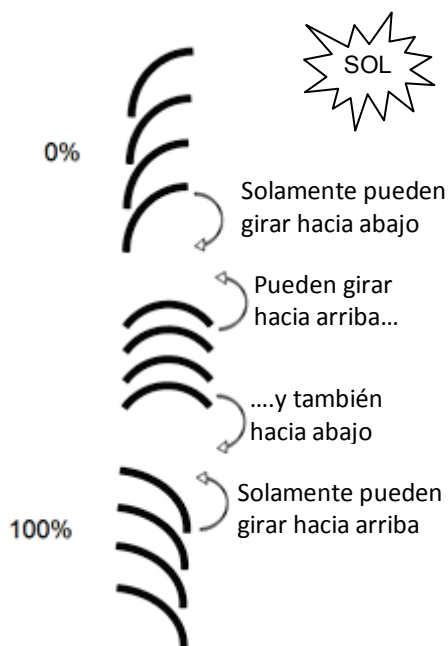
Figura 20. Posiciones "arriba" y "abajo" de las lamas
