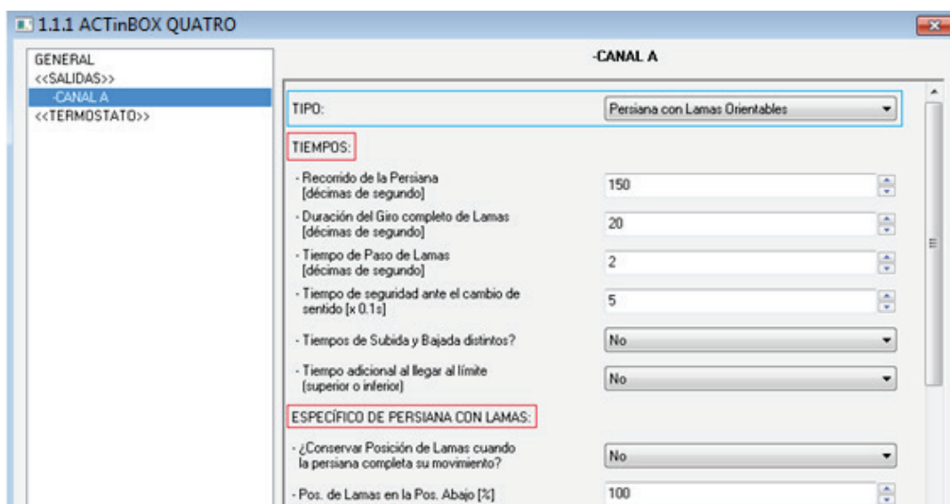
Figura 21. Pantalla de configuración de persiana con lamas en ETS
