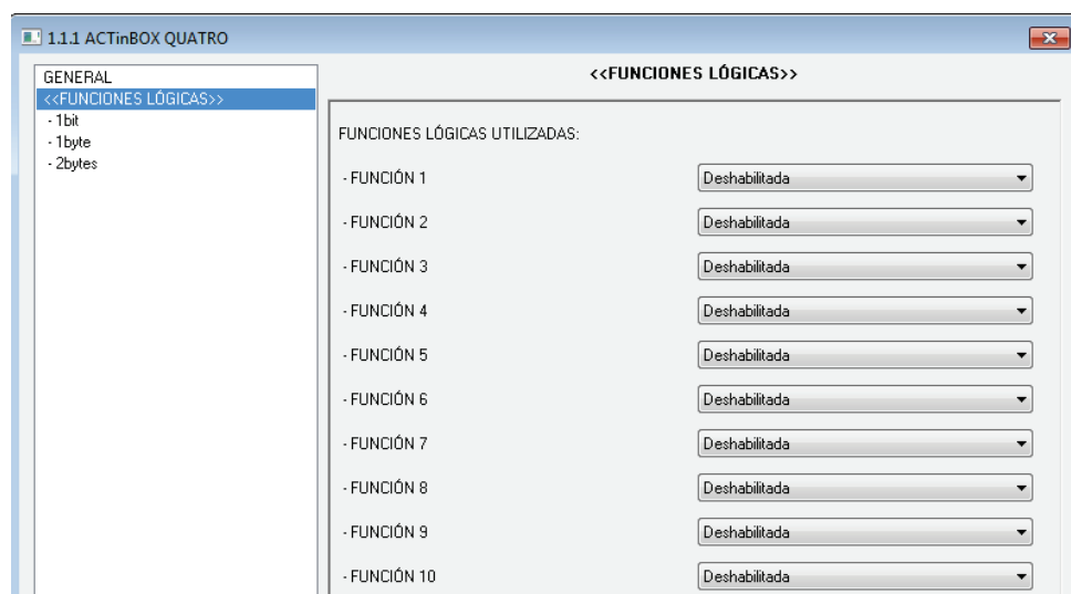
Figura 19. Pantalla de funciones lógicas
