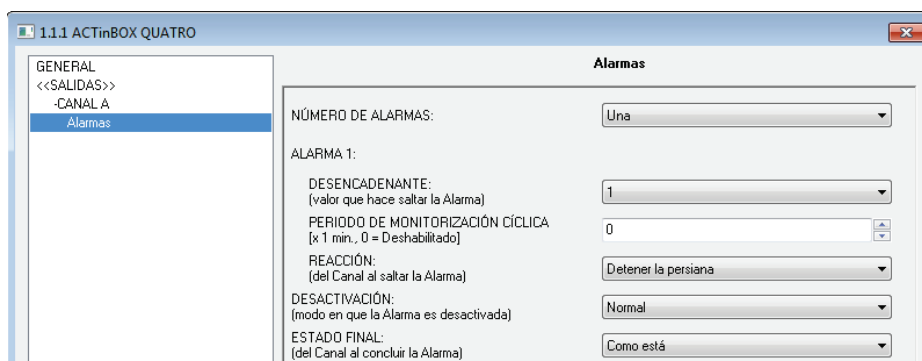
Figura 16. Pantalla de alarmas
