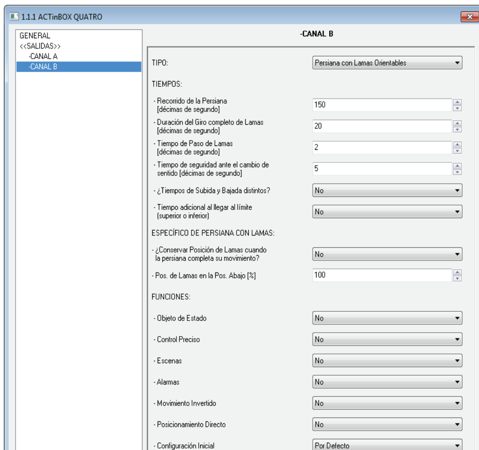
Figura 14. Canal B configurado como canal de persiana de lamas orientables
