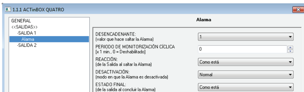
Figura 11. Pantalla de alarma
