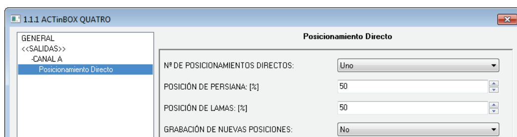
Figura 17. Pantalla de posicionamiento directo
