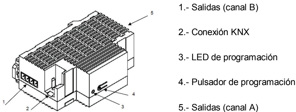
Figura 2. ACTinBOX QUATRO. Esquema de elementos
