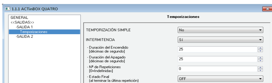
Figura 9. Pantalla de temporizaciones. Intermitencia
