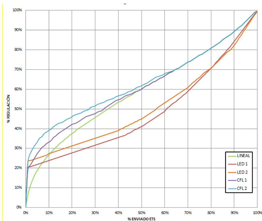
Figura 6 Curvas de regulación para cargas led y CFL.
