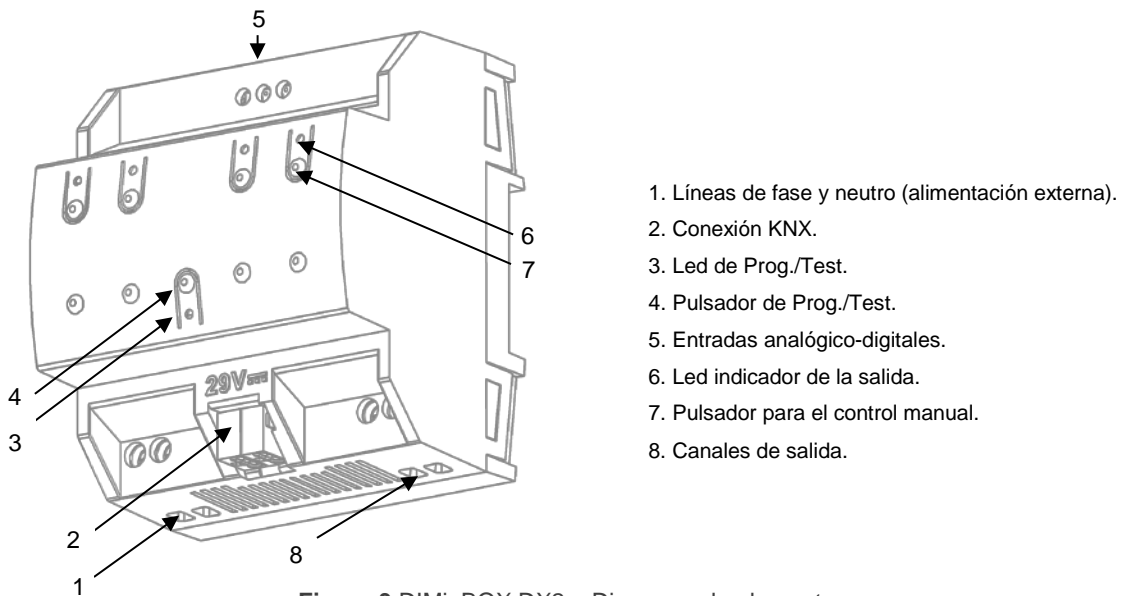
Figura 3 DIMinBOX DX2 – Diagrama de elementos.
