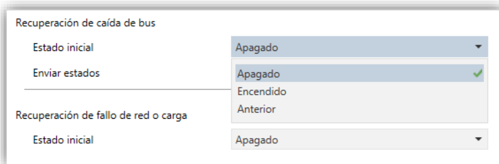
Figura 23 Inicialización.
