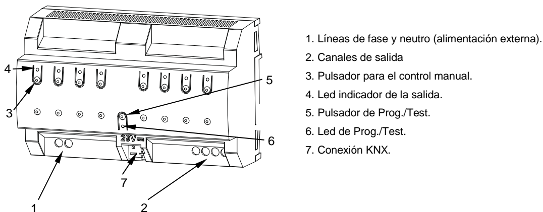
Figura 4 DIMinBOX DX4 – Diagrama de elementos.
