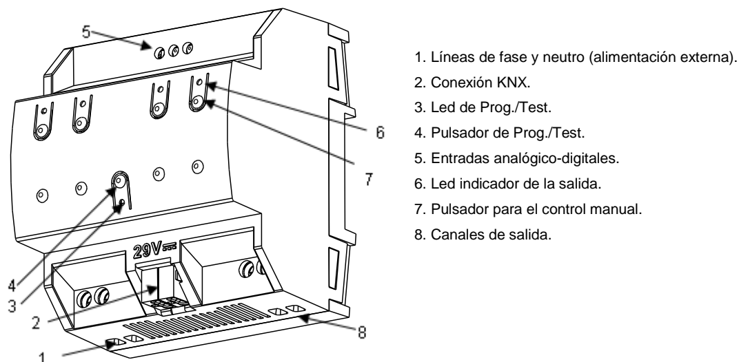
Figura 3 DIMinBOX DX2 – Diagrama de elementos.
