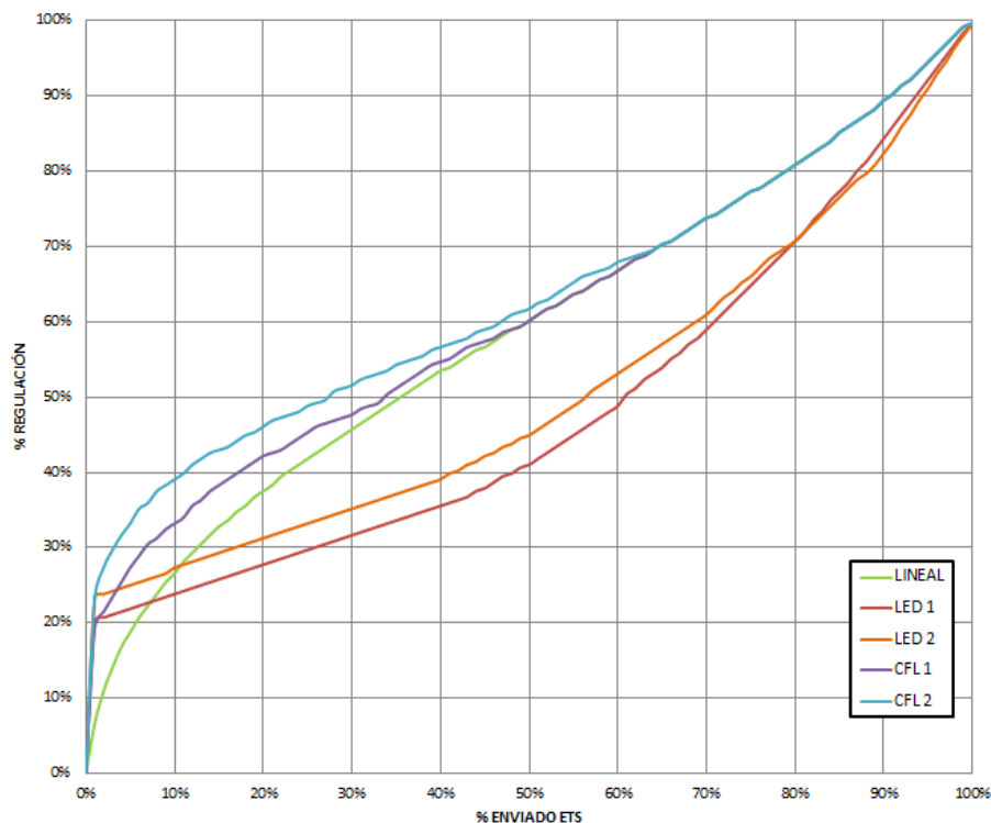
Figura 10 Curvas de regulación para cargas led y CFL.
