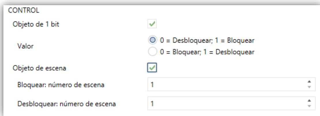
Figura 11. Bloqueo de los pulsadores: Control.
