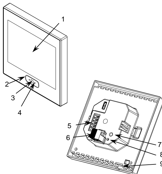
Figura 1 Diagrama de elementos.
