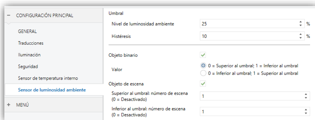
Figura 12. Sensor de luminosidad ambiente.
