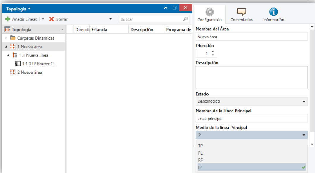
Figura 15 IP Router CL como acoplador de líneas.
