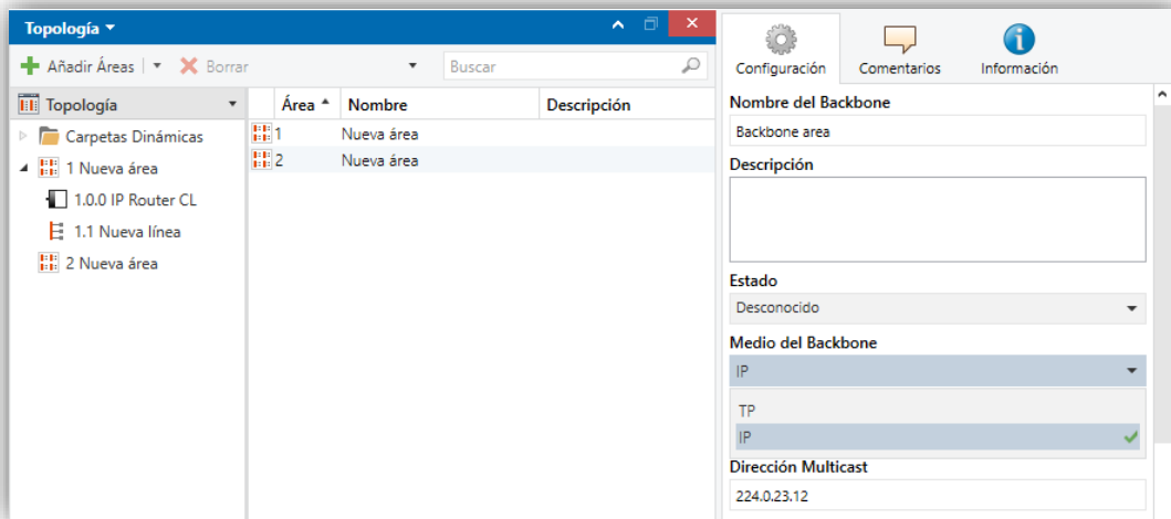
Figura 14 IP Router / Interface CL como acoplador de áreas.
