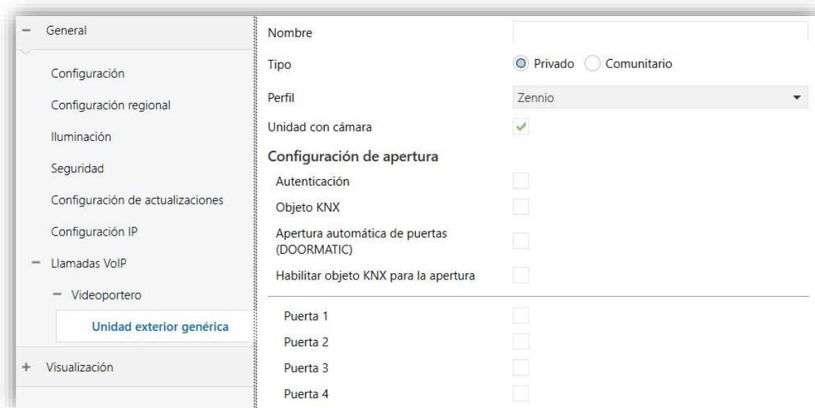
Figura 35. Unidad exterior genérica
